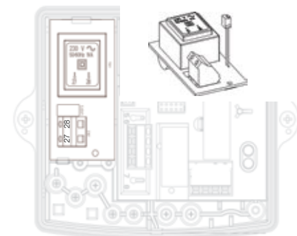
Mains module
